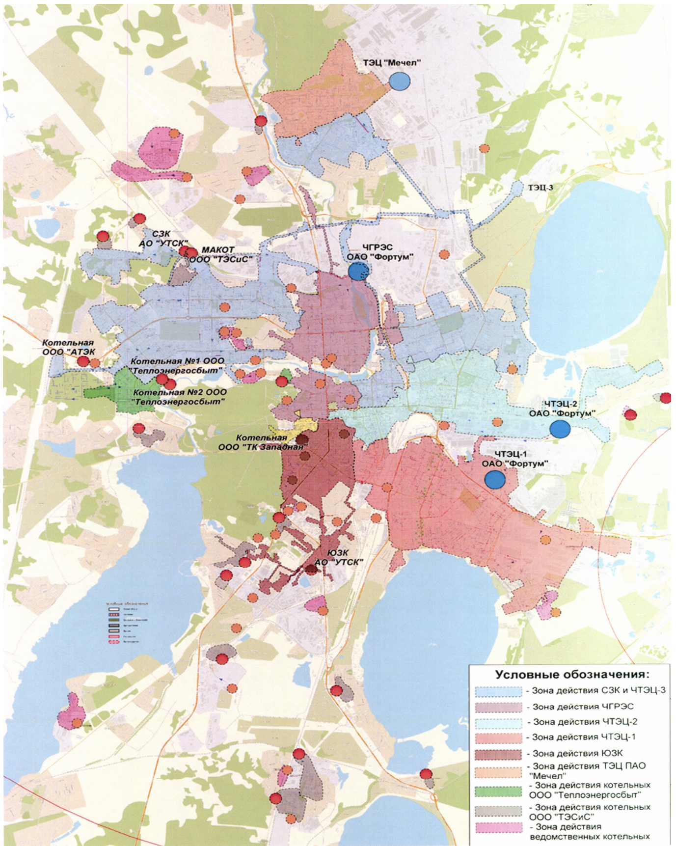
Рисунок П1.1. Зоны деятельности единой теплоснабжающей организации
