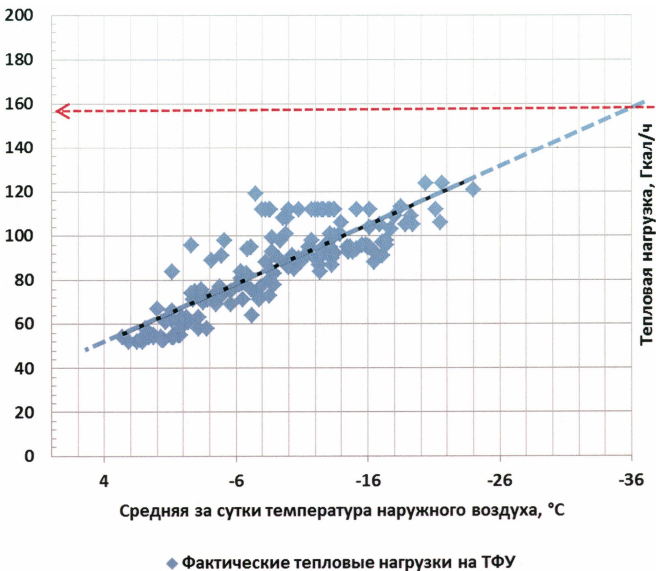
Рисунок П14.1. Определение расчетной тепловой нагрузки
