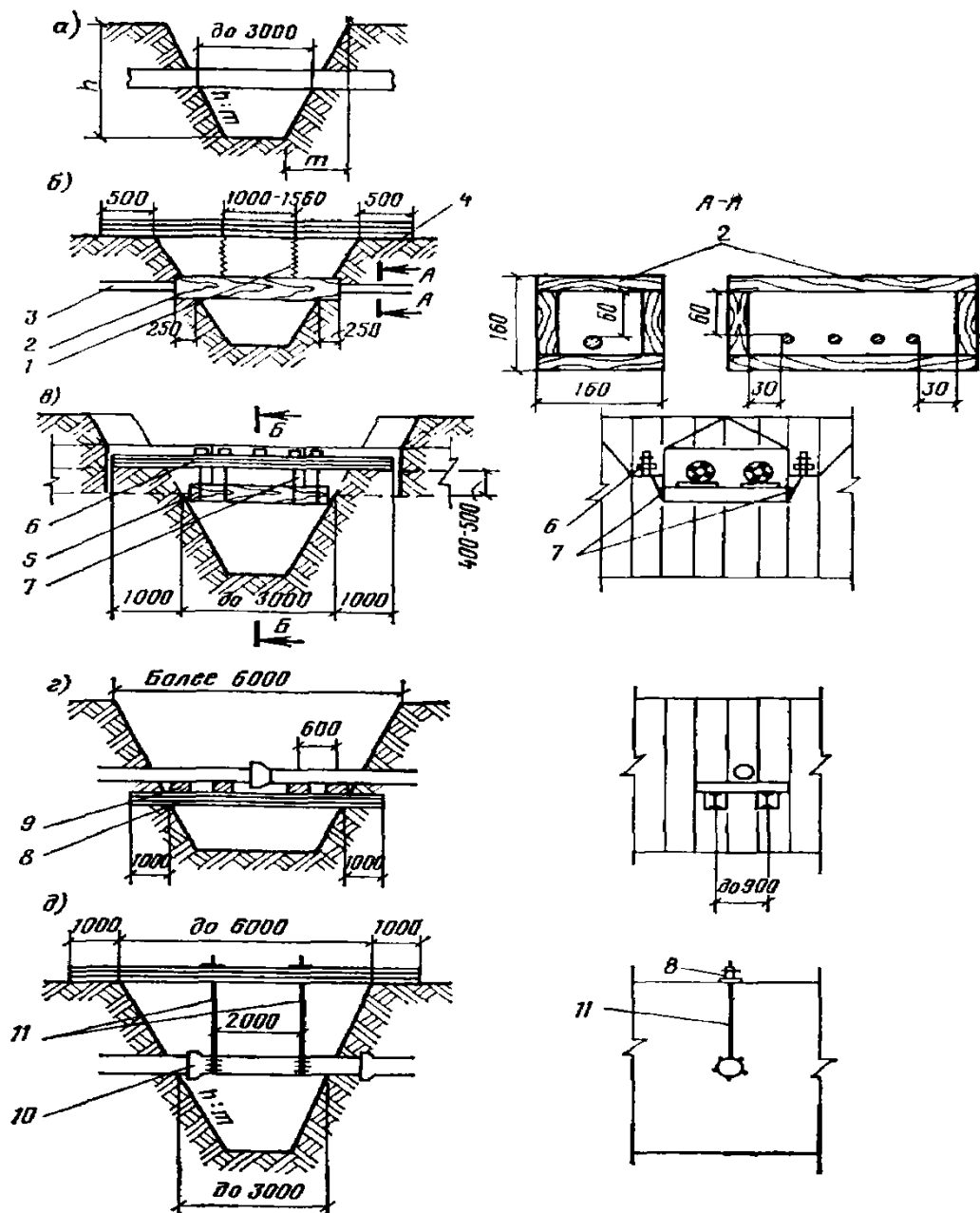
Рисунок 7.8 – Защита вскрываемых инженерных систем от механических повреждений:
