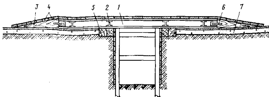
Рисунок 7.9 – Временный мост для автомобильной дороги:
