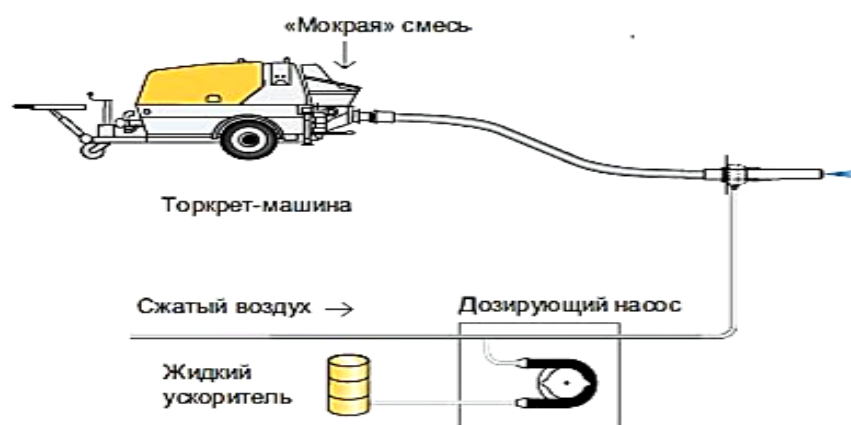
Рисунок 10.2 – Схема мокрого способа пневмобетонирования (торкретирования)
