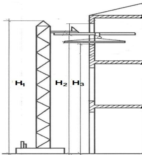
Рисунок 10.6 – Монтаж конструкций через проемы здания
