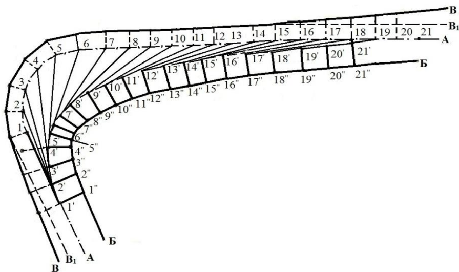
Рисунок Н1 – Построение кривой вписываемости автомобильных транспортных средств
