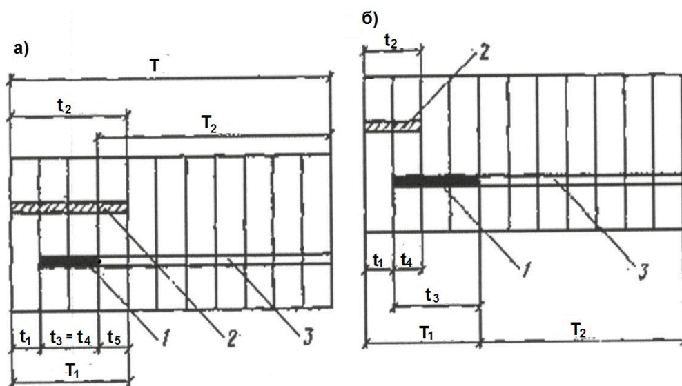
Рисунок 7.3 – Принципиальная организационно-технологическая схема производства работ:
