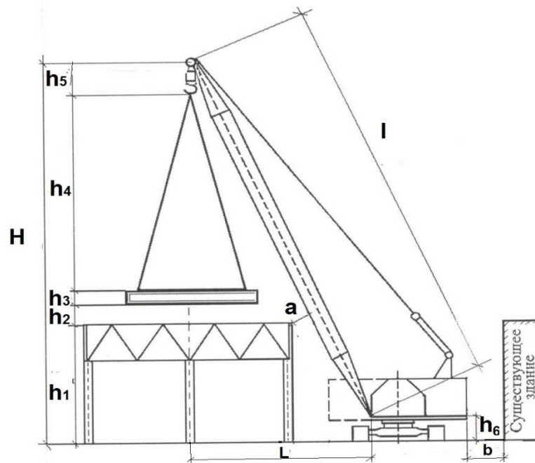
Рисунок 10.5 – Монтаж конструкций, выполняемый через верх здания
