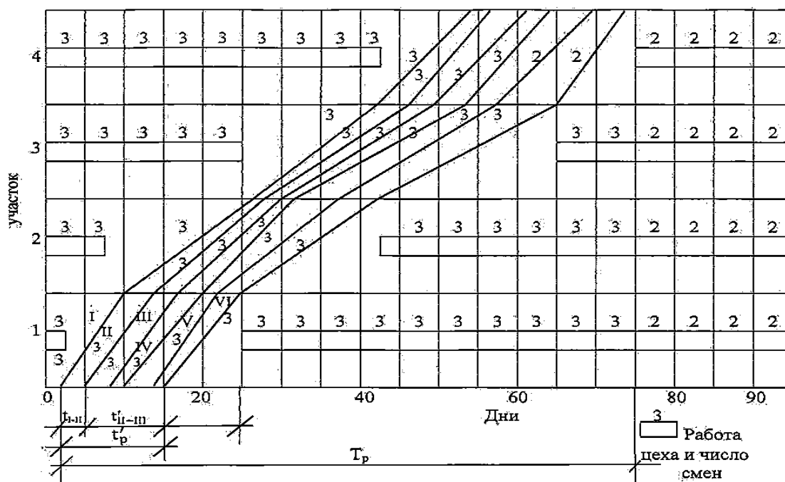
Рисунок 4.1 – Пример графика потока при реконструкции цеха с частичной остановкой производства. Вариант с поочередной остановкой производства на реконструируемых участках: I–VI – специализированные потоки, 1, 2, 3 – количество смен работы
