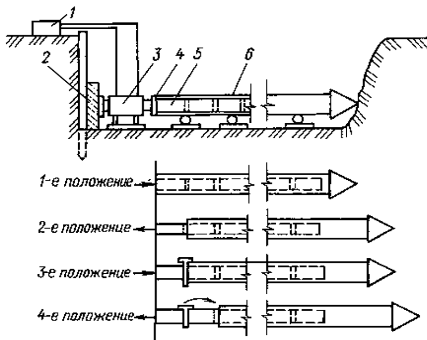
Рисунок 7.12 – Схема прокладки трубопроводов способом прокола:
