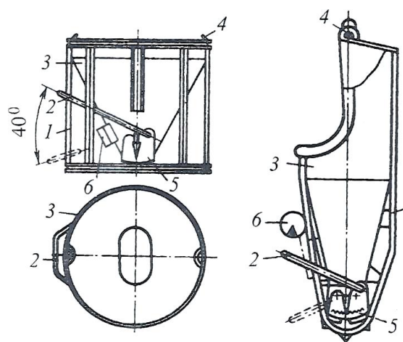
Рисунок 10.1 – Бункеры (бадью) для бетонной смеси:
