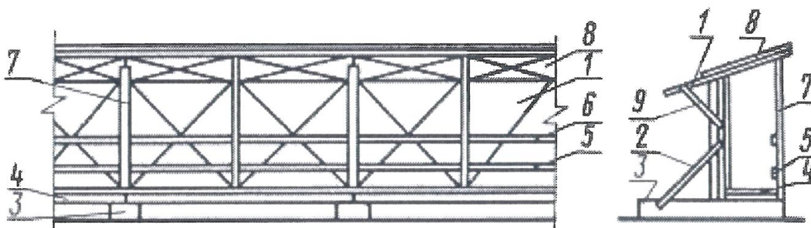
Рисунок 7.2 – Схемы ограждений:
