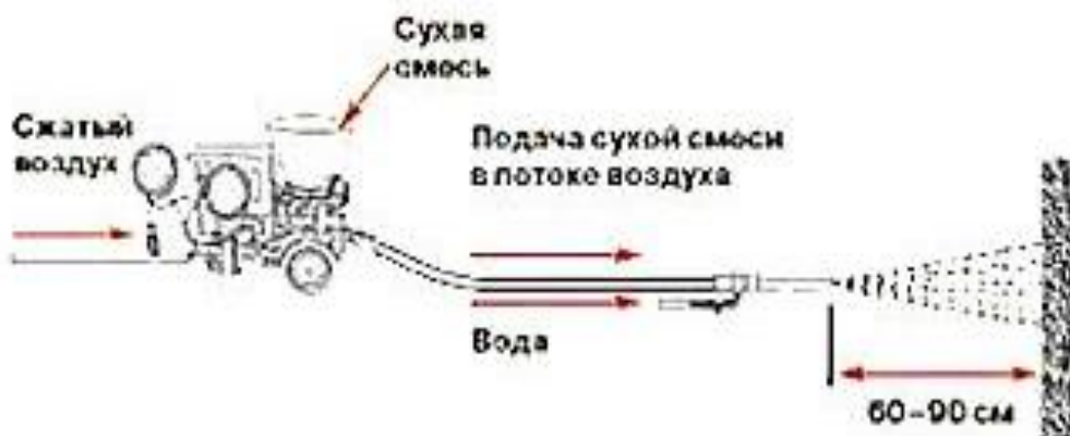
Рисунок 10.3 – Схема сухого способа пневмобетонирования (торкретирования)
